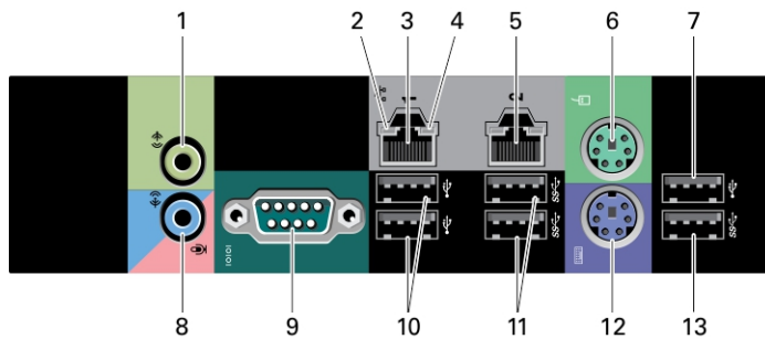
Ilustración 4. Vista del panel posterior
