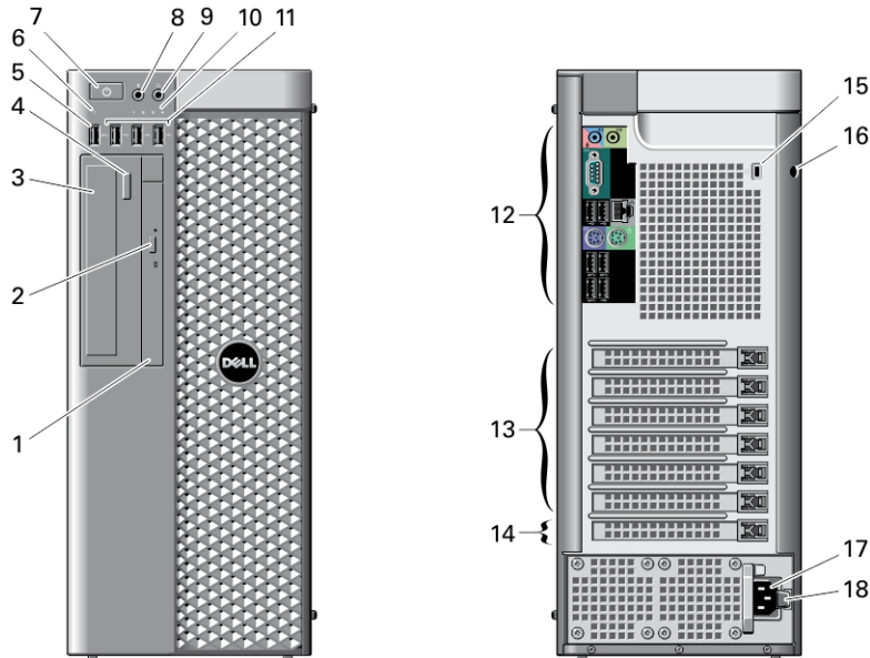
Ilustración 1. Vistas frontal y posterior de T3610/T5610
